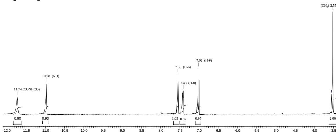
Рисунок 2.23. Спектр ЯМР ^1\text{H} 7-бром-1,5-дигидро-2Н-хромено-[2,3- d ]пиримидин-2,4(3 H )-диона
