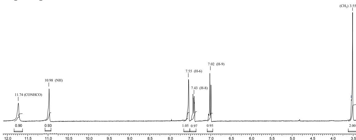
Рисунок 2.23. Спектр ЯМР ^1\text{H} 7-бром-1,5-дигидро-2Н-хромено-[2,3- d ]пиримидин-2,4(3Н)-диона
